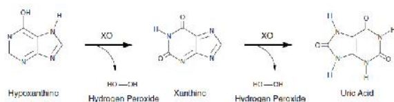
Gambar 1. Mekanisme Konversi Xantin Menjadi Asam Urat
